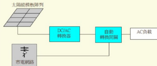
典型併聯式太陽光電能系統
