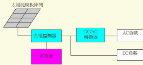
供應交/直流負載之獨立式太陽光電能系統
